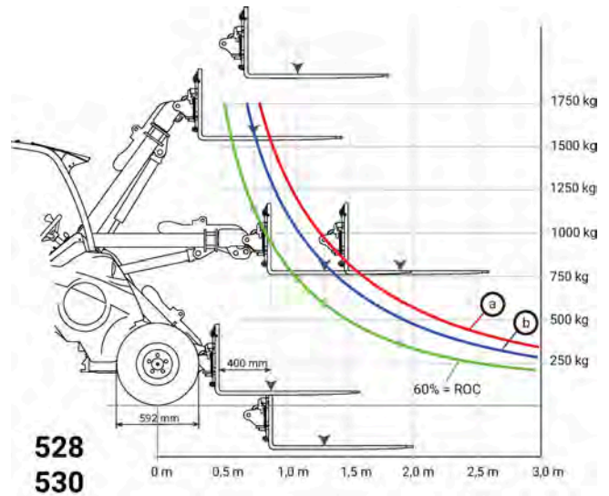
Diagram zaťaženia 528 & 530
